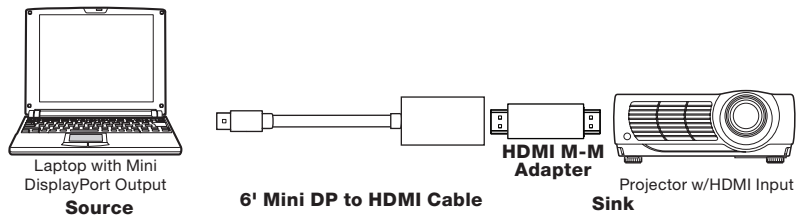
Mini DP-HDMIF/6 with HDMI M-Male coupler 26-679-06
